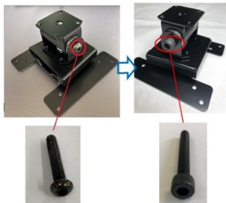
キャップボルト
