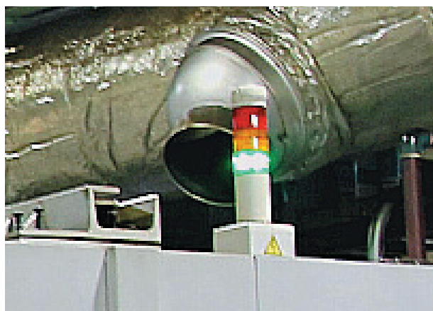
加工設備に設置されているパトライト表示灯とAirGRID®の設備
