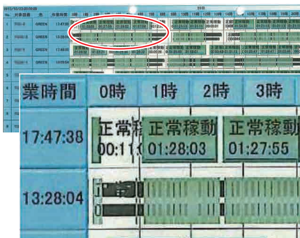
ガントチャートによる可視化例(サイクルタイムを可視化)
