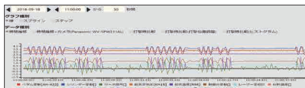
各種センサデータの時系列分析
